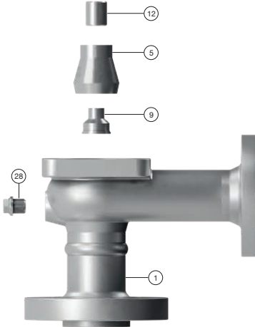
Explosionszeichnung ES
