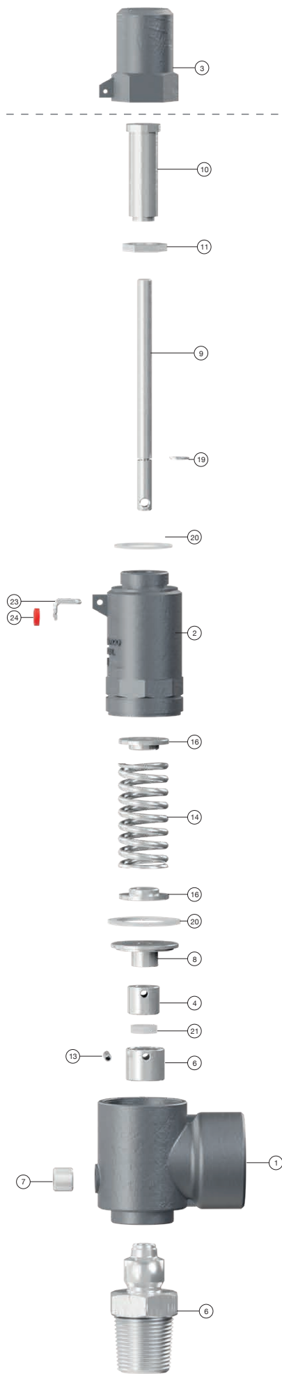
Despiece ES
